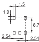
Actual Mounting Pad Dimensions
