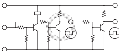
改善例②：入力と同位相の出力値が必要な場合
