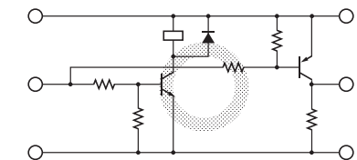
改善例②：入力と同位相の出力値が必要な場合
