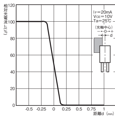
アクチュエータ設計参考図
