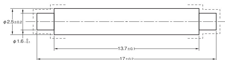
アクチュエータ設計参考図
