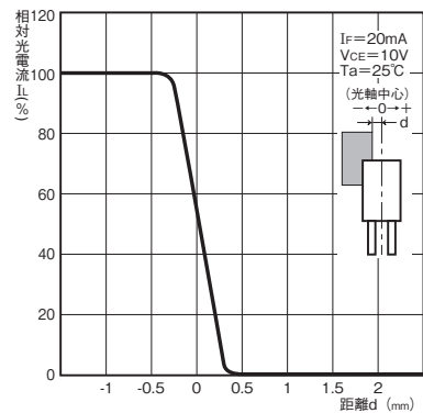
図10. 検出位置特性(TYP.) EE-SJ3-C
