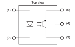
内部回路
