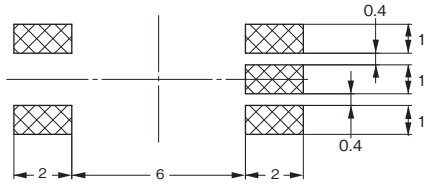
推奨はんだ付けパターン
