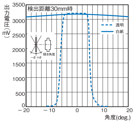
形B5W-LB2101
