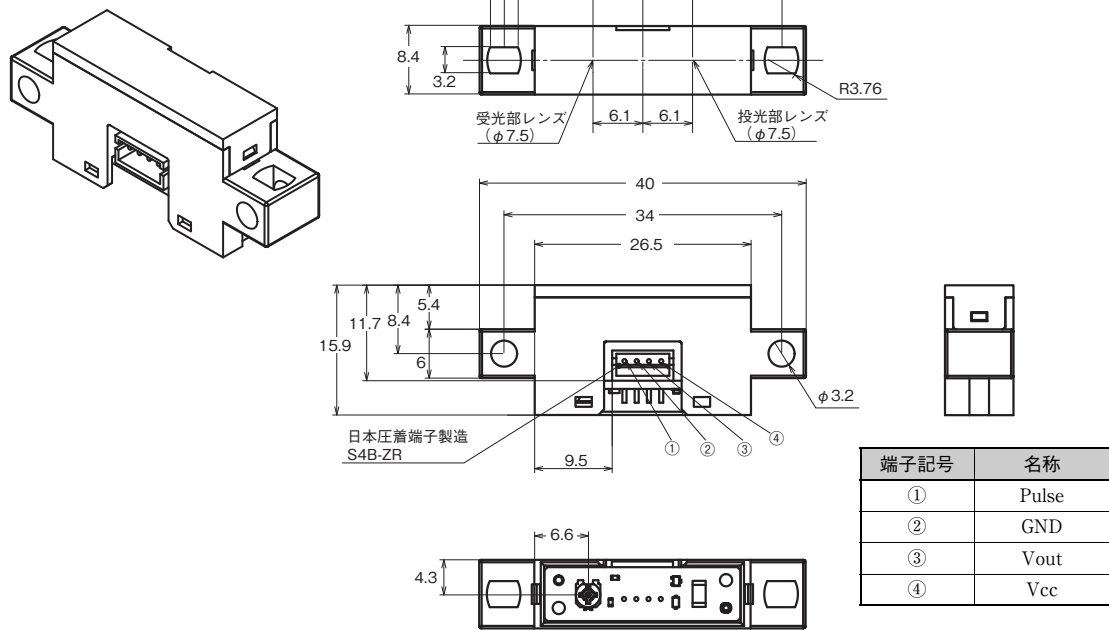
形B5W-LB2101-1
