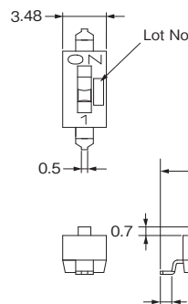
1極スイッチ外形寸法図
