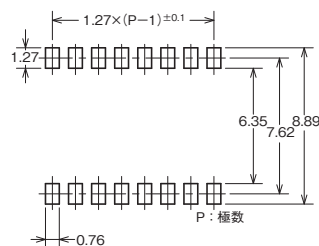
プリント基板パッド寸法(参考) (TOP VIEW)
