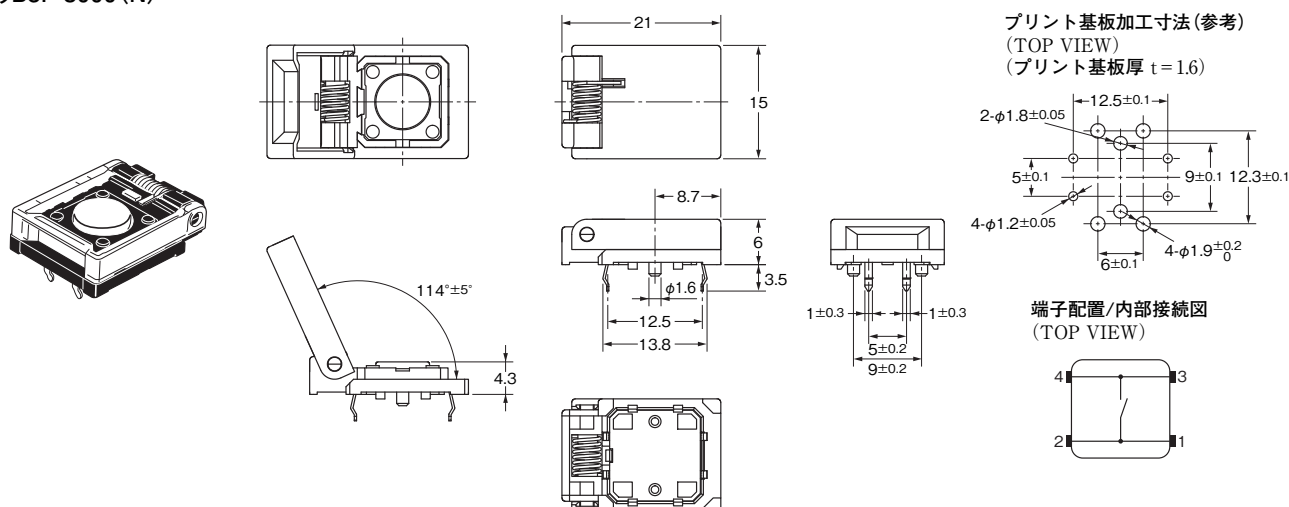
形B3F-8000(N)
