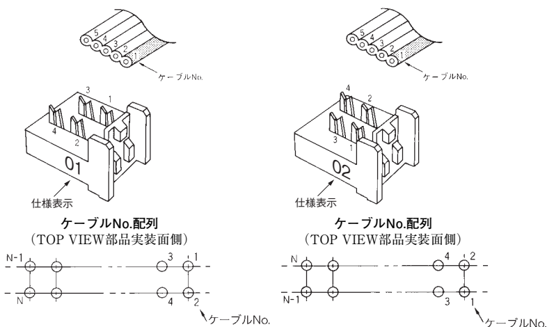
標準端子配列形
