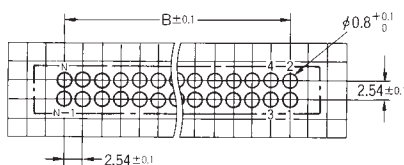
標準端子配列形の場合
