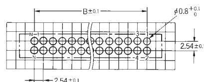
逆列端子配列形の場合
