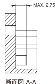
断面図 A-A
