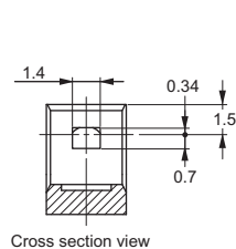
<Emitter>
