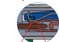
第1ばね 挿抜時・かん合時 接触 第2ばね 挿抜時 開放 かん合時 接触力印加
