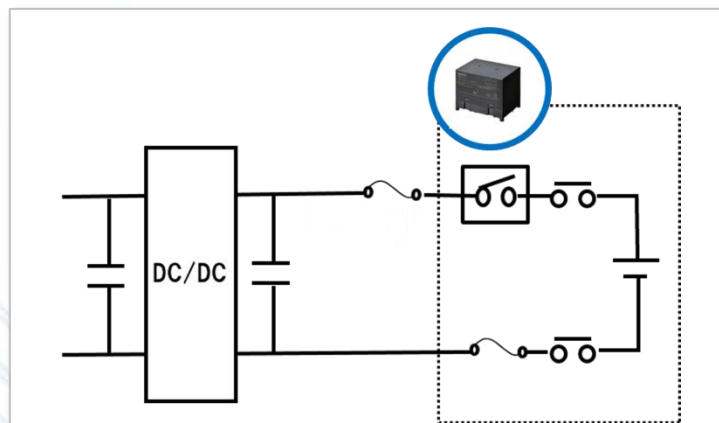
図18: 電力貯蔵用途の例
