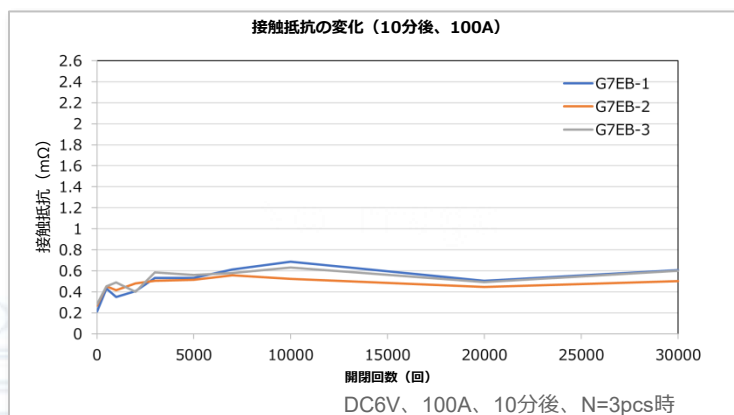
図5: 接触抵抗の変化（参考データ）
