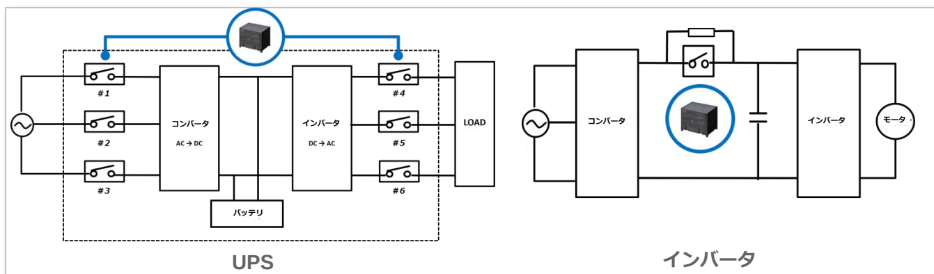
図3: 商用および産業用UPSと産業用インバータでの使用例
