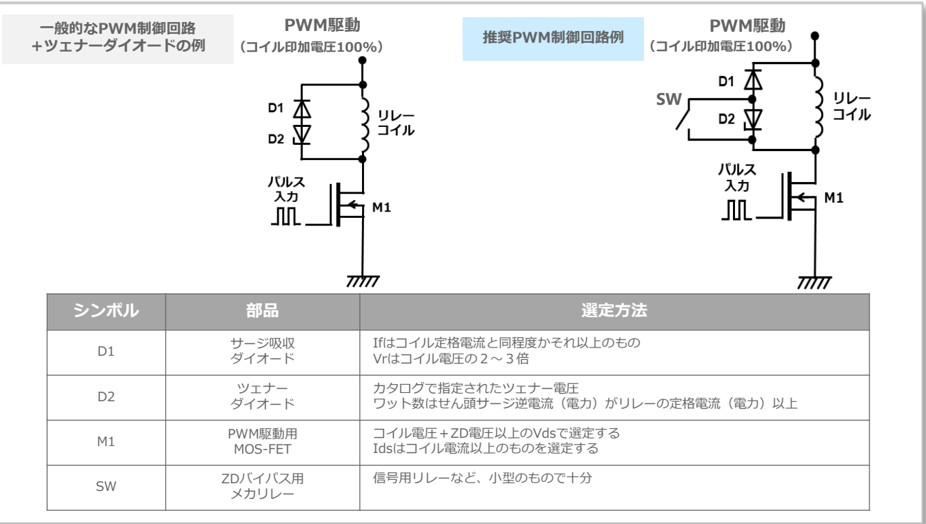
図15: PWM制御回路の参考図
