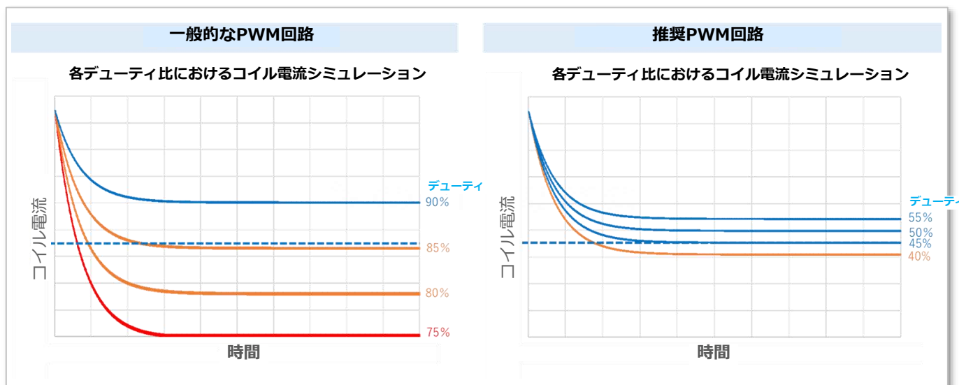
図17: PWM制御時の電流推移
