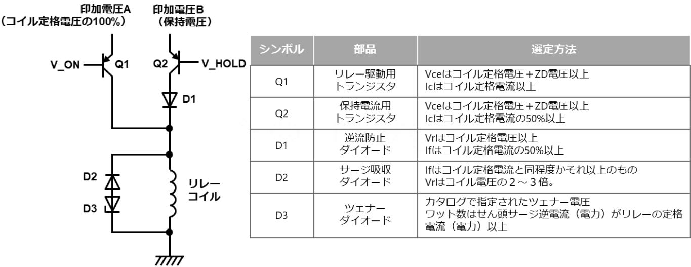
図13:スイッチによる推奨保持電圧回路例、周辺部品の選定方法
