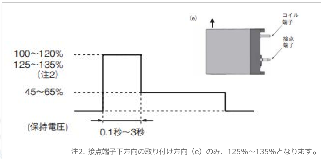
図8: 保持電圧
