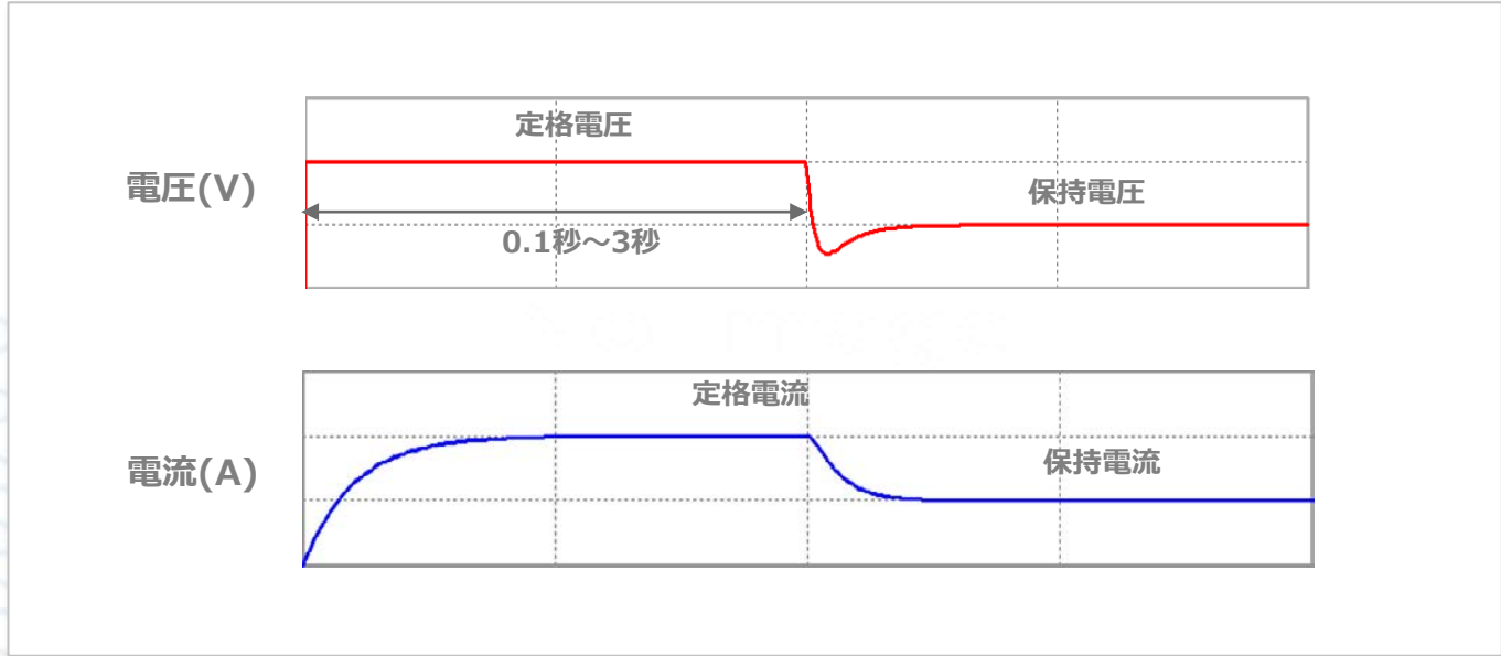
図10:CR回路におけるコイル電圧・電流波形例
