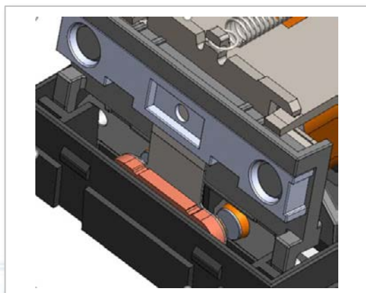
図19: G7EBシリーズの接点構造
