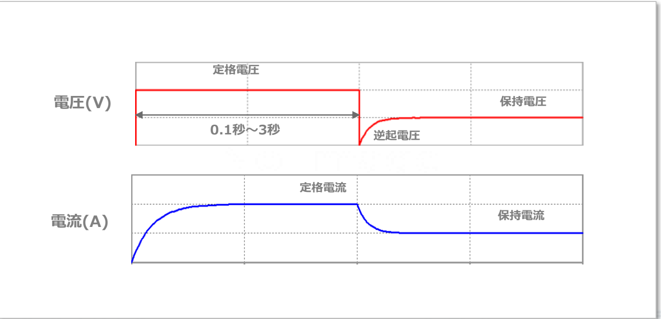
図12:スイッチによる保持回路におけるコイル電圧・電流波形例
