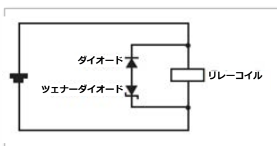
図7: ダイオード接続
