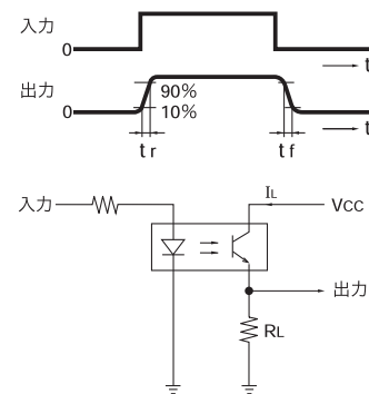
図9. 応答時間測定回路
