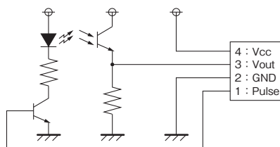
内部回路
