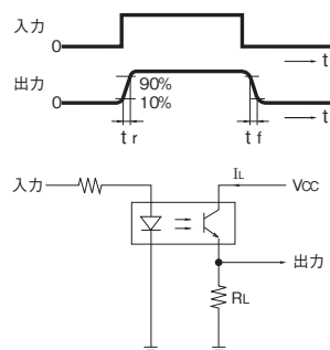
図10. 応答時間測定回路
