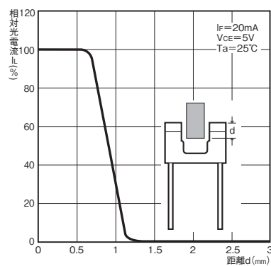
図9. 検出位置特性(TYP.)
