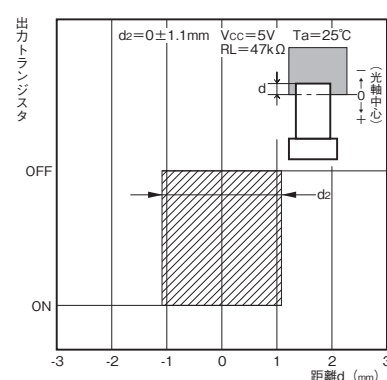
図3. 検出位置特性 (TYP.)
