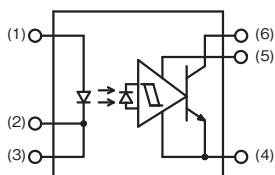
内部回路
