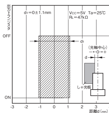
図2. 検出位置特性 (TYP.)
