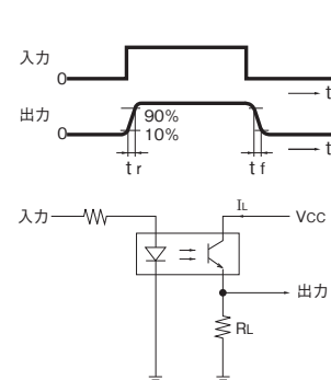
図12. 応答時間測定回路
