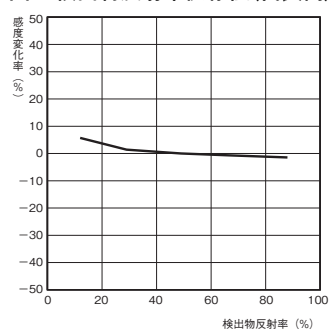
図2. 検出物反射率依存性(代表例)
