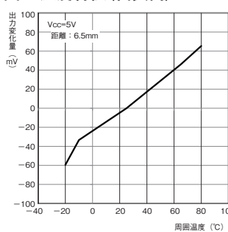
図3. 温度特性(代表例)
