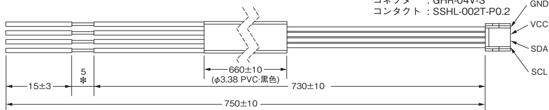
ケーブル : UL1061.AWG#28 CADデータ
