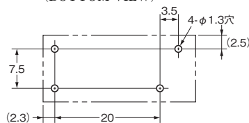
プリント基板加工寸法 (BOTTOM VIEW)
