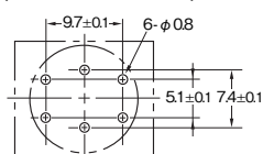
プリント基板加工寸法 (BOTTOM VIEW)
