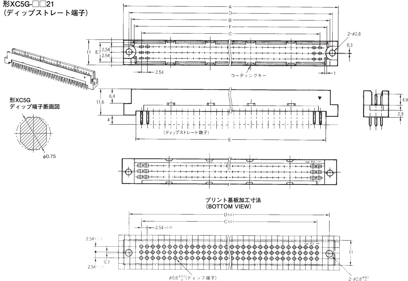
寸法表
