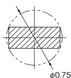
形XC5B ディップ端子断面図
