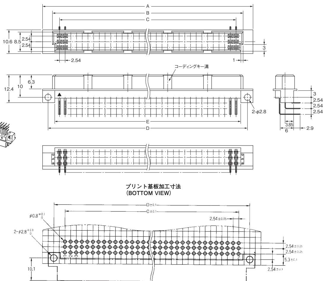
寸法表
