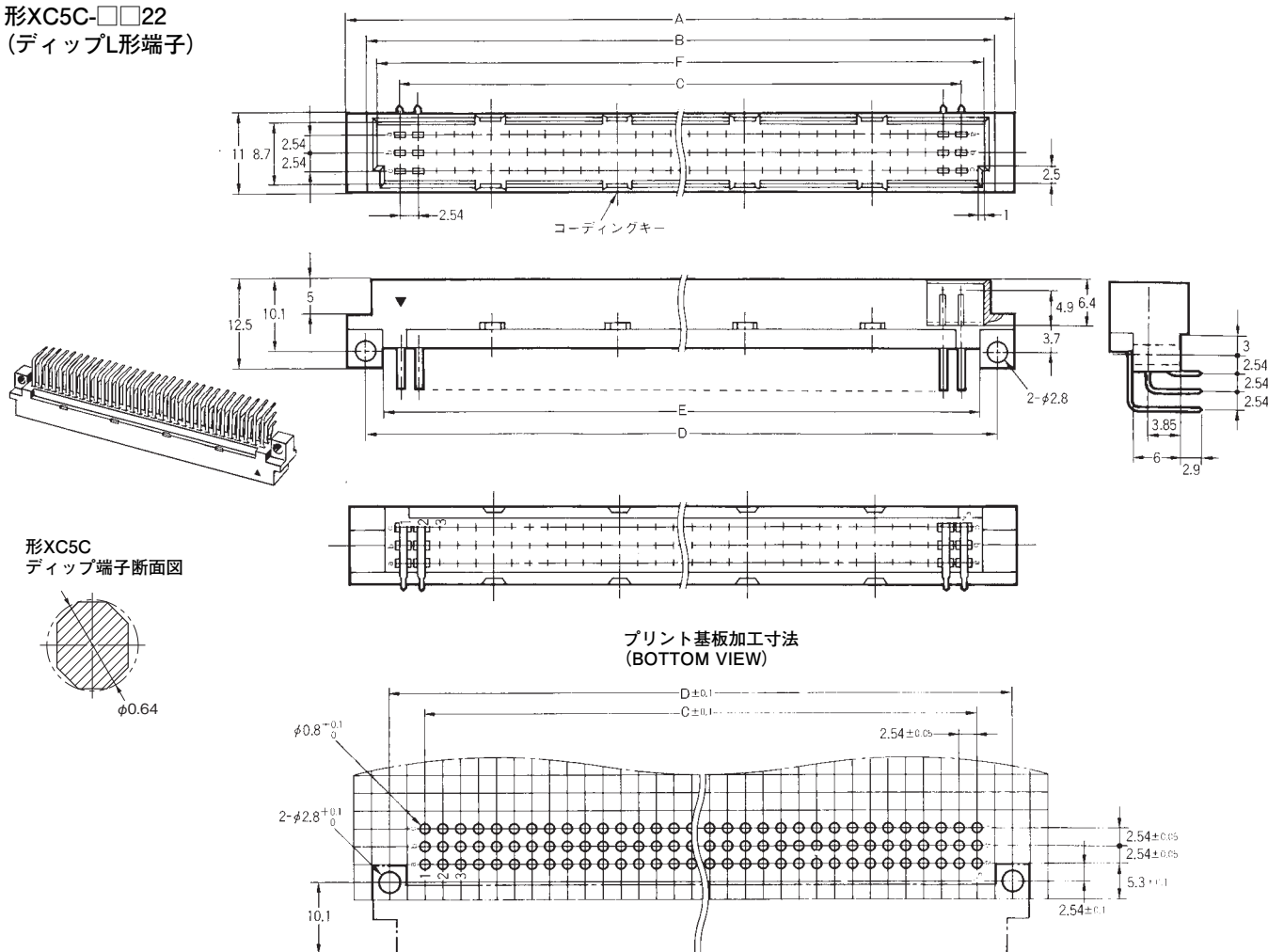
寸法表
