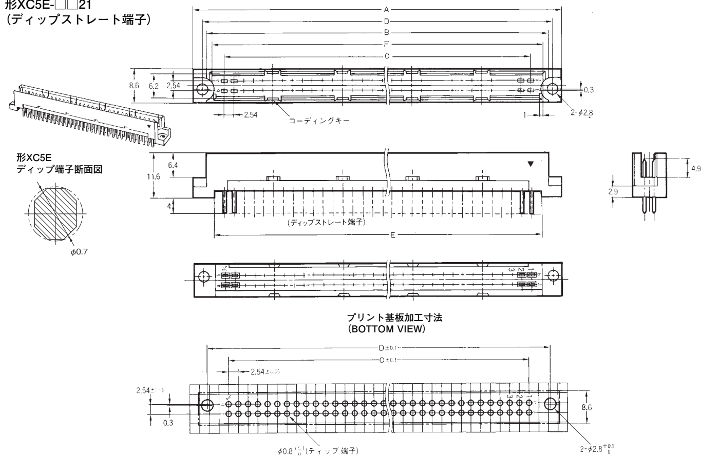
寸法表
